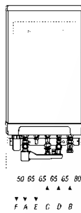
Conexiones hidráulicas salida inferior con plantilla
