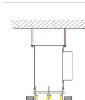
Montaje con Plenum
