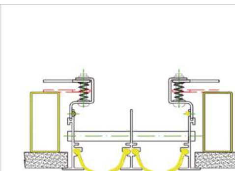
Montaje con pestillos
