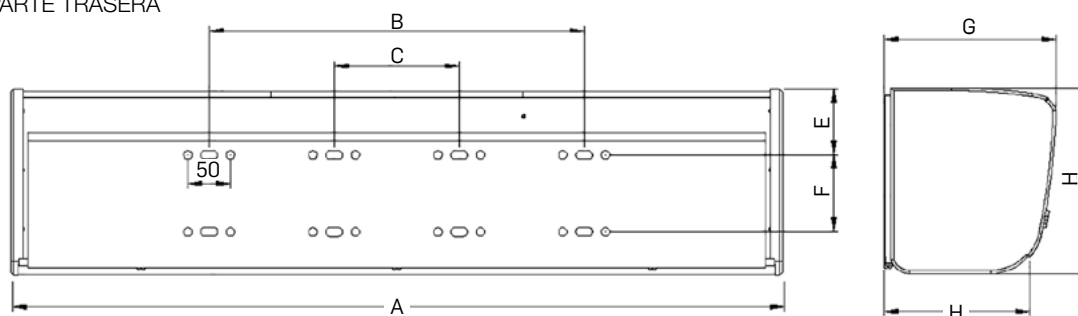
PARTE TRASERA
